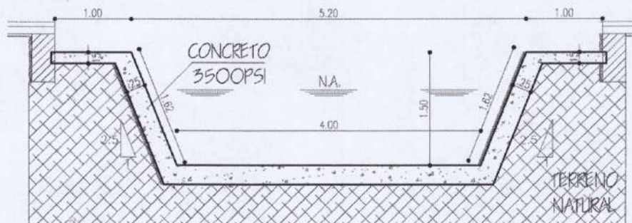
Ilustración 10. Sección del Canal Trapezoidal en Concreto Proyectado en el Arroyo del Barrio 11 de abril 7 .
