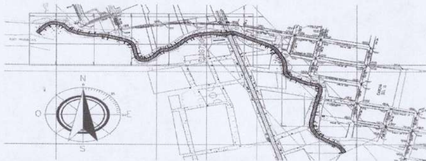
Ilustración 9. Tramo de canal trapezoidal en concreto proyectado en el Arroyo del Barrio 11 de abril 6 .
