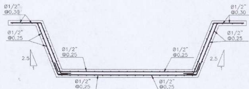
Ilustración 11. Despiece del acero de refuerzo del canal en concreto proyectado.
