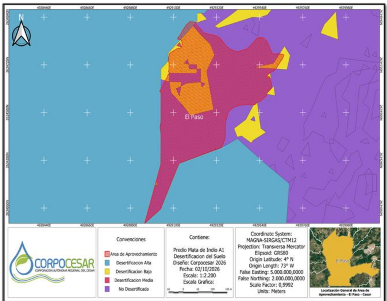
Imagen 5. Superposición de árboles aislados en predio MATA DE INDIO 1B y Desertificación del Suelo. Fuente CORPOCESAR 2026.
