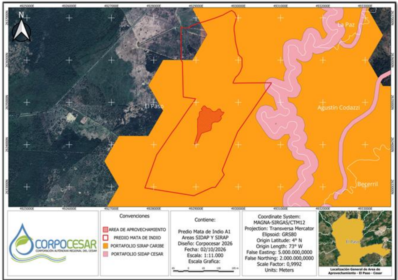
Imagen 6. Superposición de árboles aislados en predio MATA DE INDIO 1B, Área de aprovechamiento y Areas SIDAP y SIRAP. Fuente CORPOCESAR 2026.
