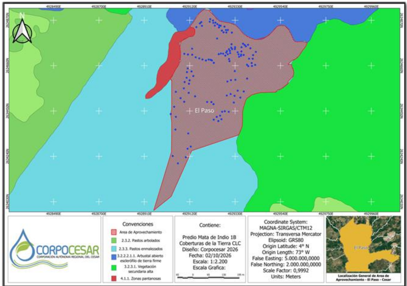
Imagen 7. Superposición de árboles aislados en predio MATA DE INDIO 1B, Área de aprovechamiento y Cobertura de la tierra CLC 1:25.000 año 2022. Fuente CORPOCESAR 2026.
