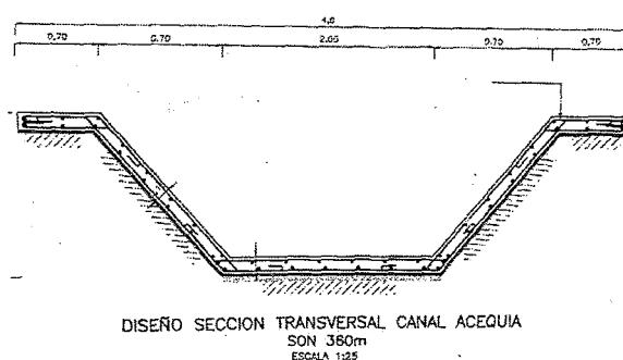
Imagen 11. Diseño de la sección transversal del cauce Fuente: Propia
